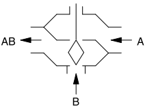
Смесительный клапан
